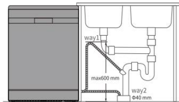
Lắp độc lập
