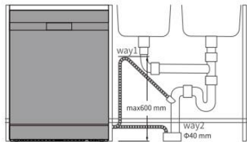
Lắp vào khoang tủ bếp (bỏ nắp trần)
